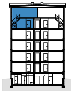
PRZEKRÓJ
