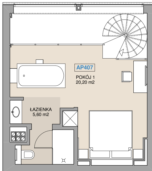
POZIOM 1- 25,80m 2
