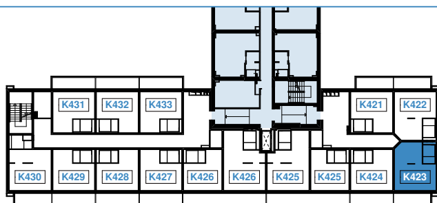
RZUT PIĘTRA 4
