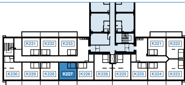
RZUT PIĘTRA 2
