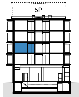
PRZEKRÓJ
