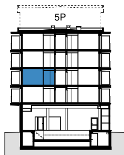
PRZEKRÓJ
